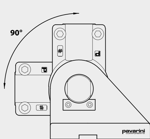
ACCOPIAMENTO IKB CON TAPR...CE ASSEMBLING IKB WITH TAPR...CE
