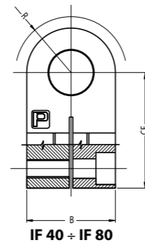
IF 40 + IF 80
