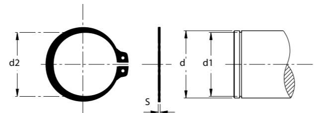
TIPO - TYPE A DIN 471 UNI 3653 - 7435
